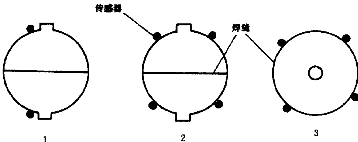
图 B1 气瓶用传感器阵列布置图
