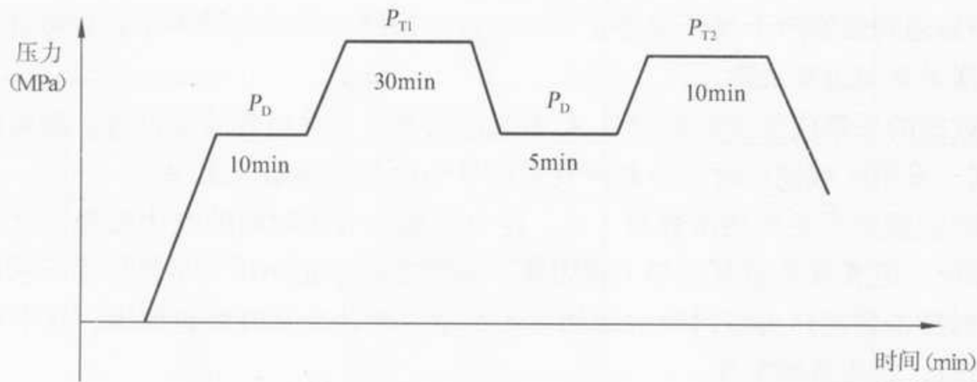
图1 在制承压设备的加压程序
