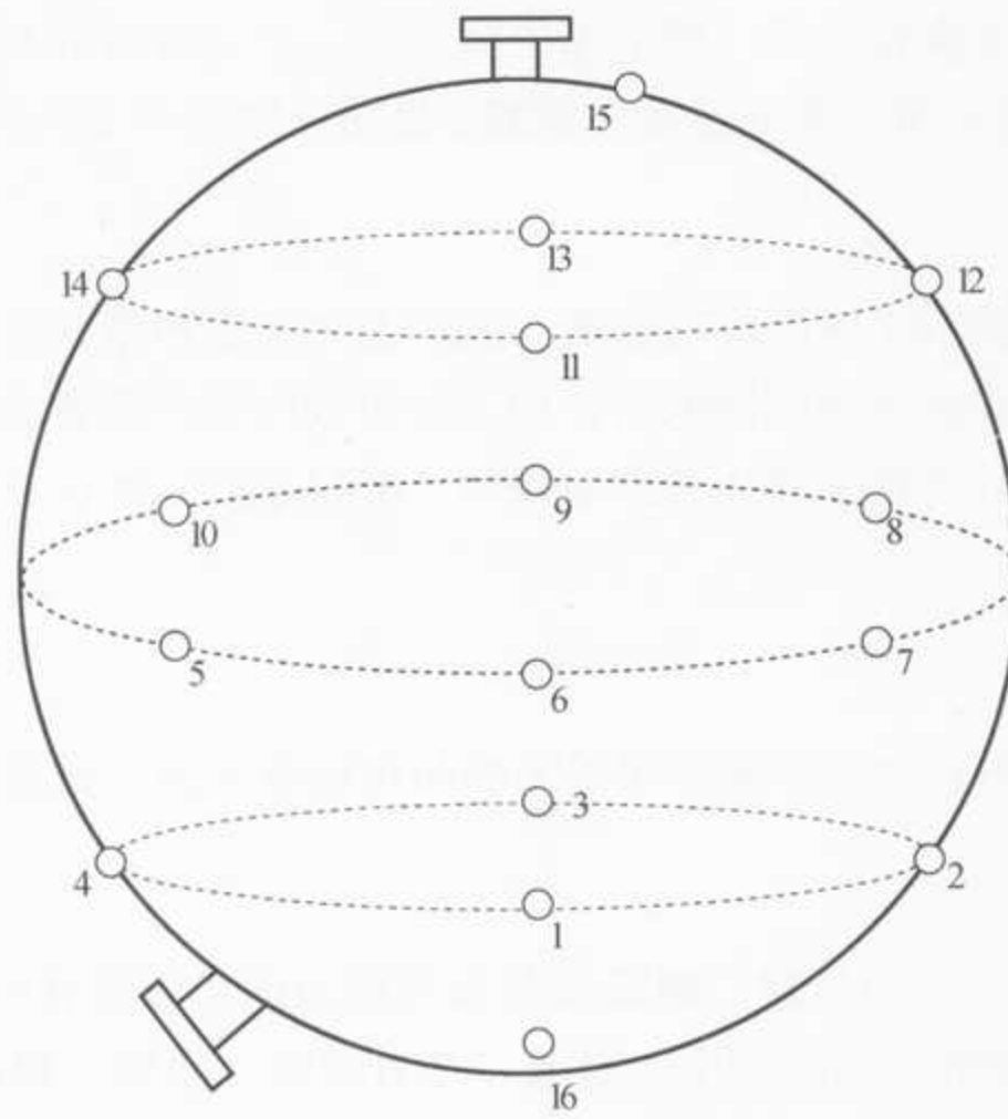
图 B.2 球形容器传感器布置示意图
